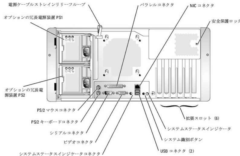
図 1-4 背面パネルのコンポーネント
